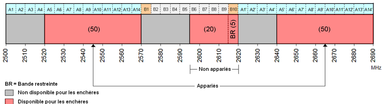
Figure C3 – Spectre disponible pour l’attribution de licences dans la région A
