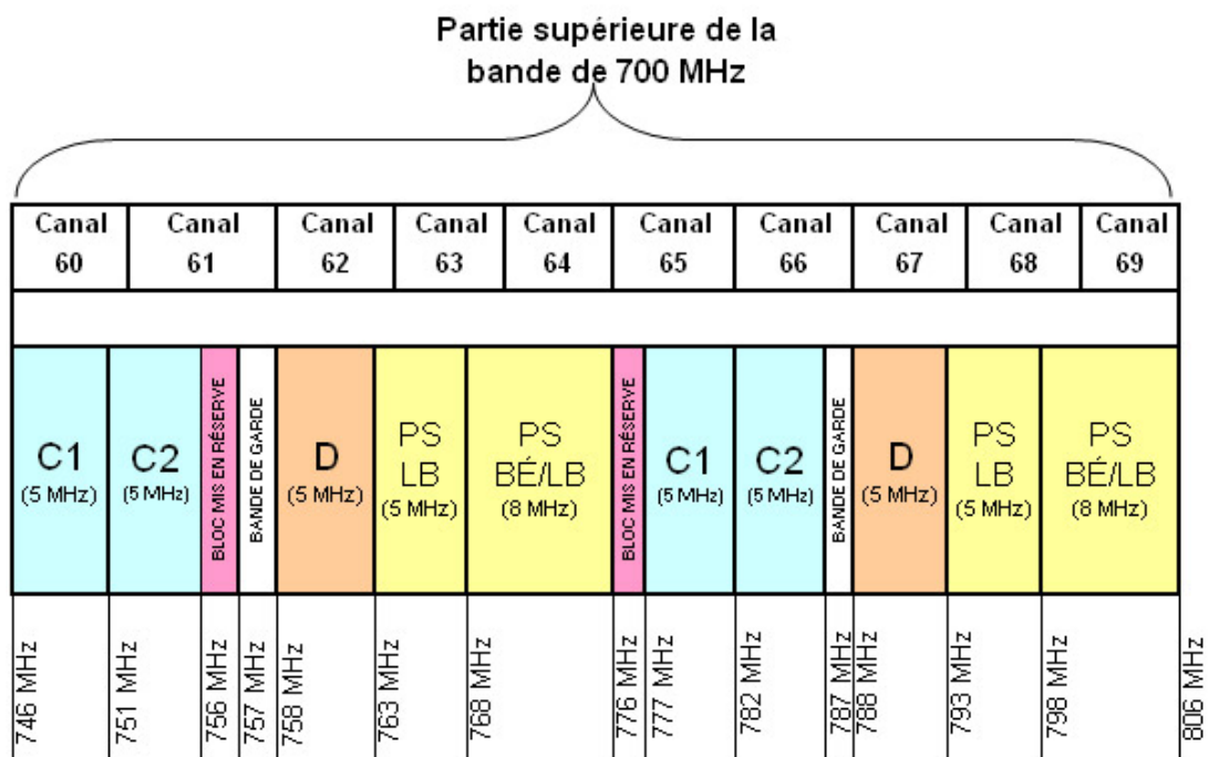
Figure B3 : Plan de répartition de la partie supérieure de la bande de 700 MHz au Canada
