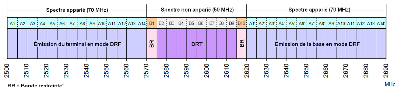
Figure C1 – Plan général pour le SRLB dans la bande 2 500-2 690 MHz
