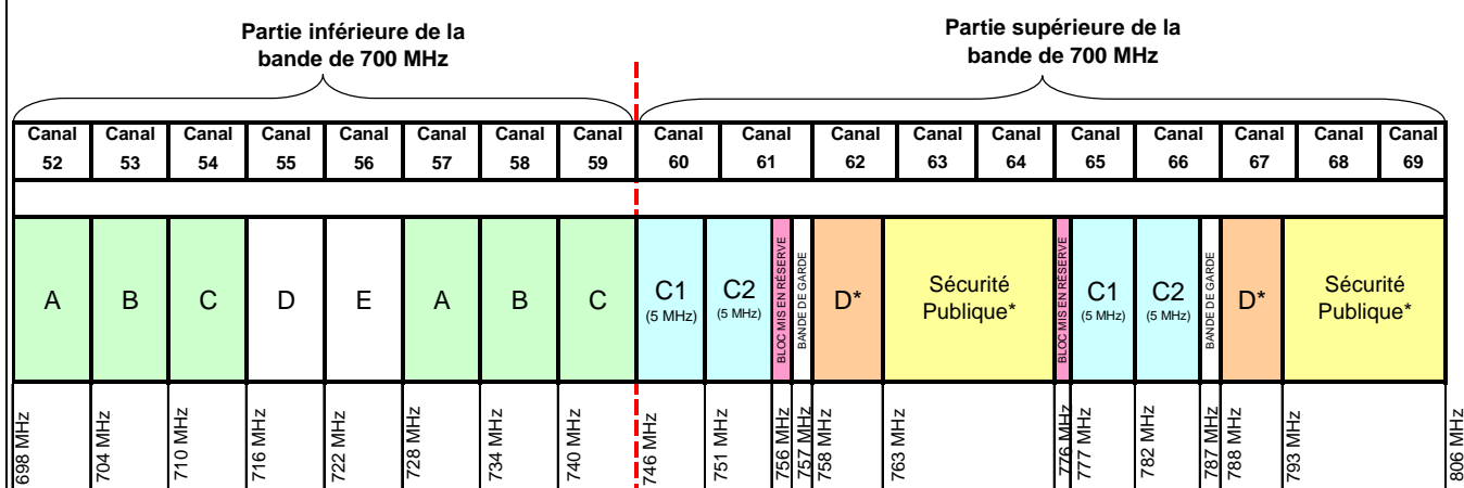
Figure B2 : Plan canadien de répartition des bandes 698-756 MHz et 777-787 MHz
