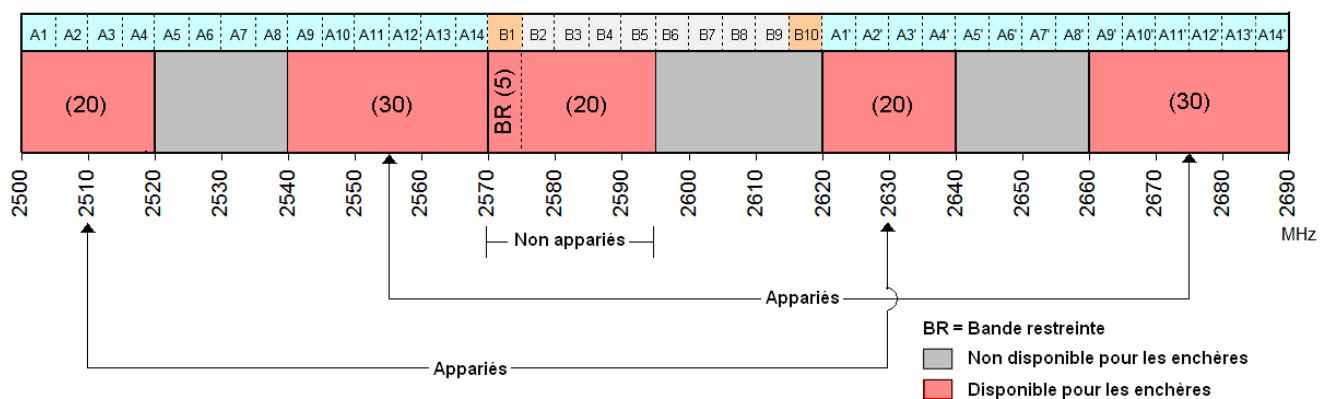
Figure C5 – Spectre disponible pour l’attribution de licences dans la région C
