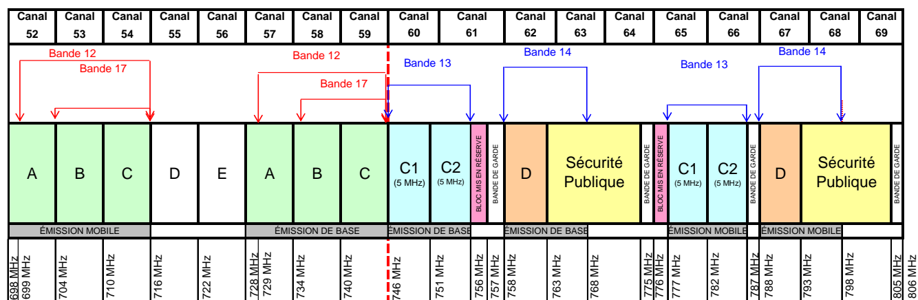
Figure B1 - Spécifications techniques élaborées par 3GPP pour le matériel fonctionnant dans la bande de 700 MHz avec la division du bloc C en deux blocs séparés
