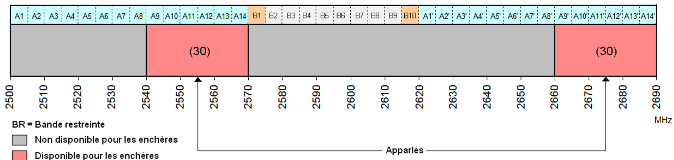
Figure C5 – Spectre disponible pour l’attribution de licences dans la région C
